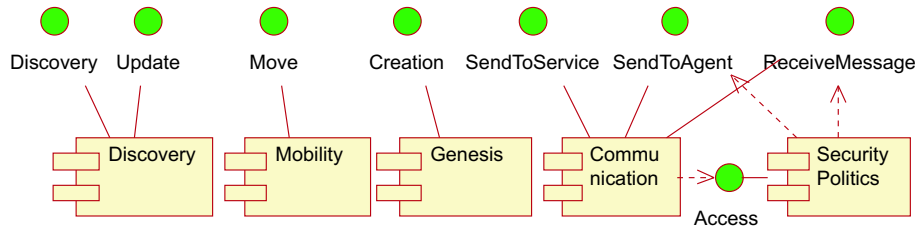
Fig. 5. BasicServices Layer
